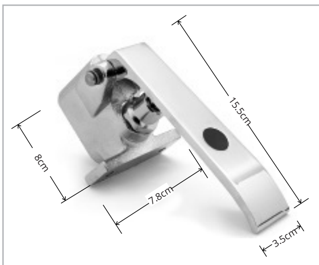
MEDIDAS DE LA VÁLVULA
